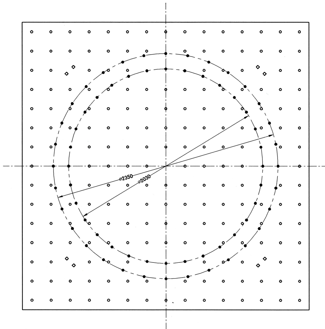
図3-6 水平振動台及び垂直振動台M12ネジ穴パターン抜粋図
