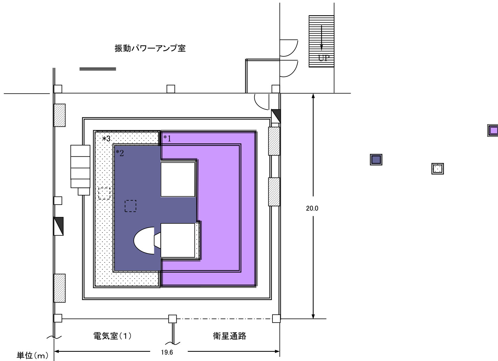
図4-4 作業床
