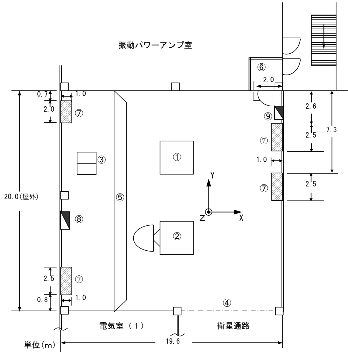
図3-1 試験室配置
