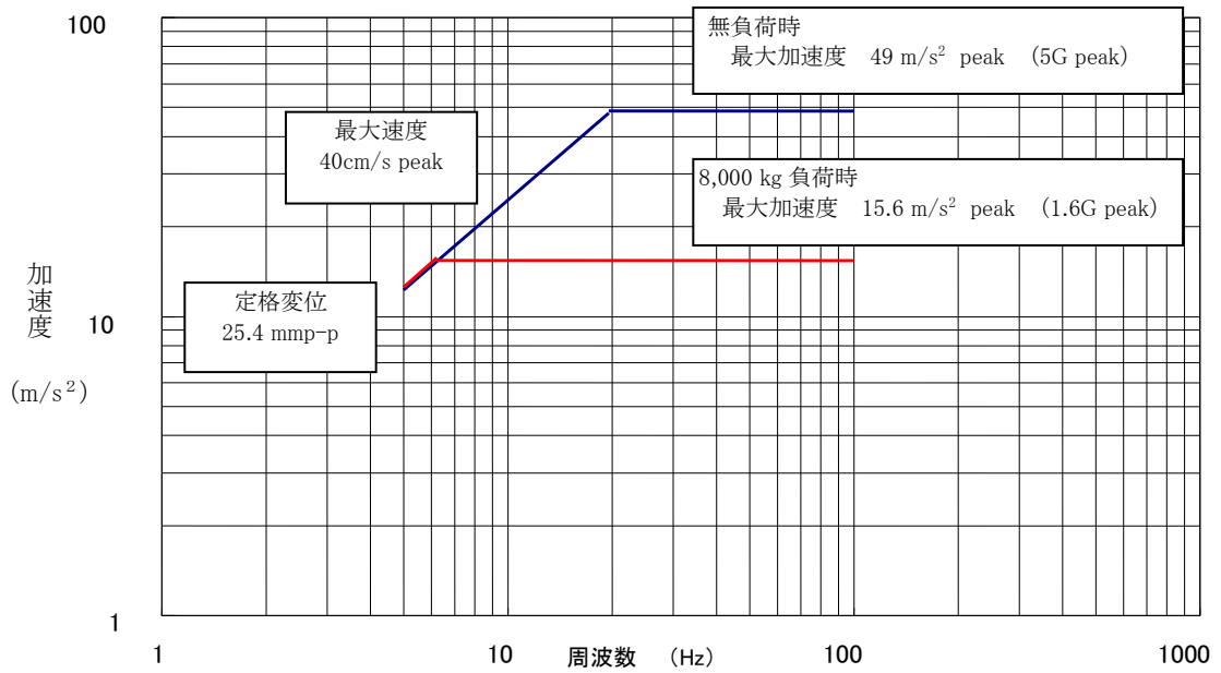
図2-4 最大加振加速度（垂直振動台）
