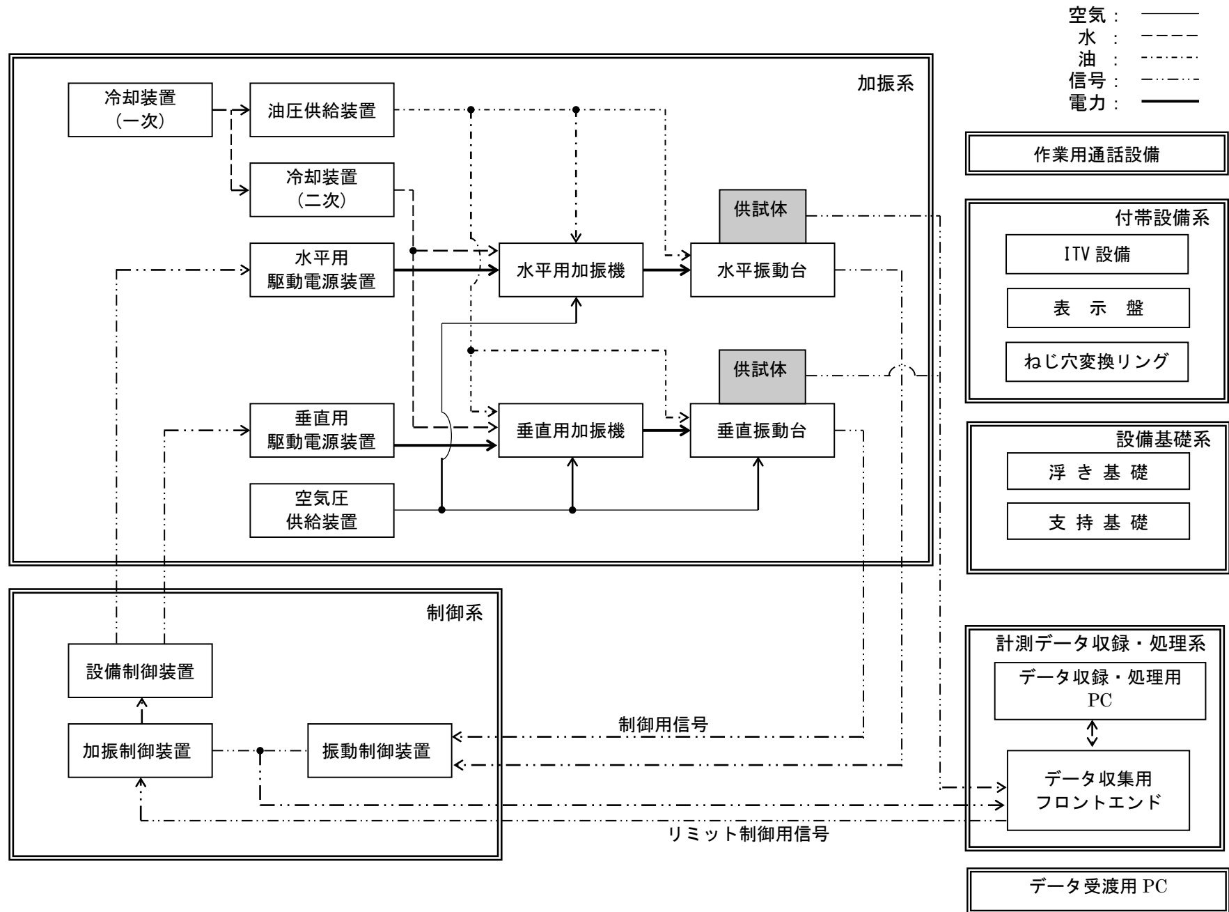
図2-2 システム構成図
