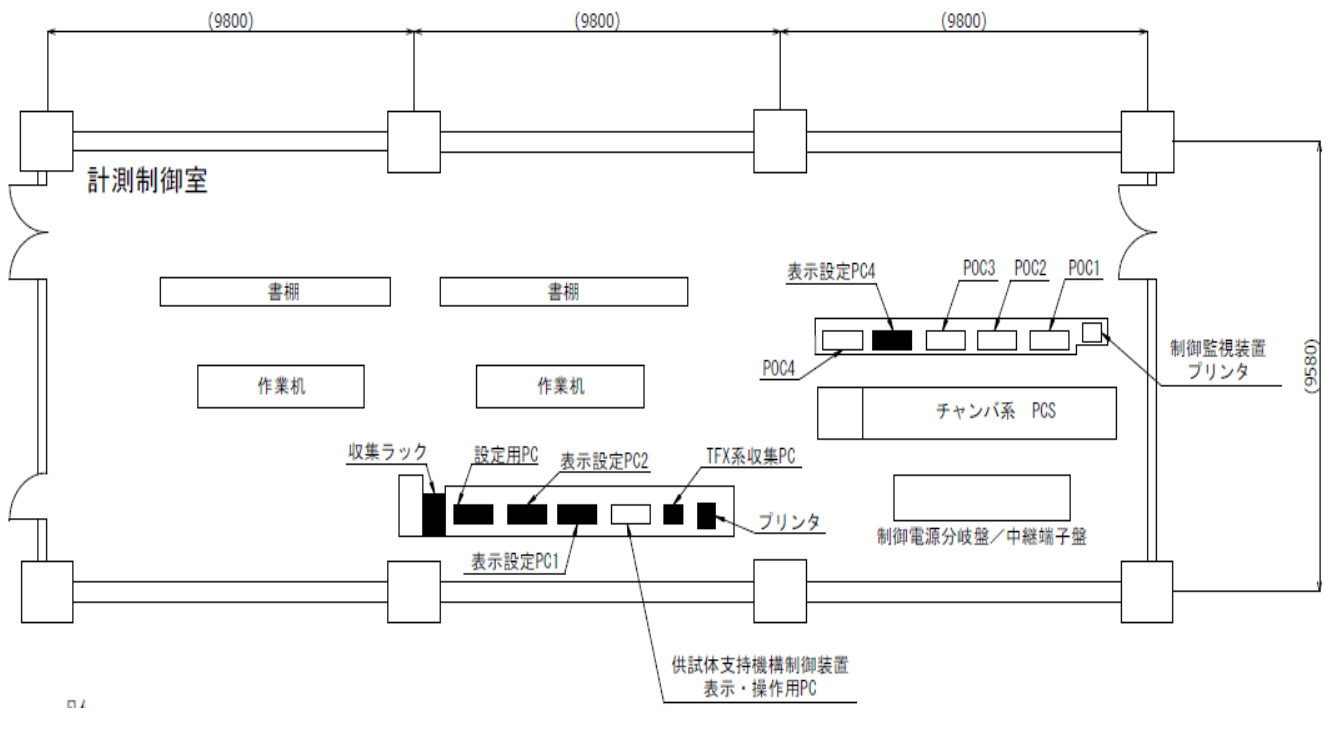
図 3-2 スペースチャンバ計測制御室（2F）
