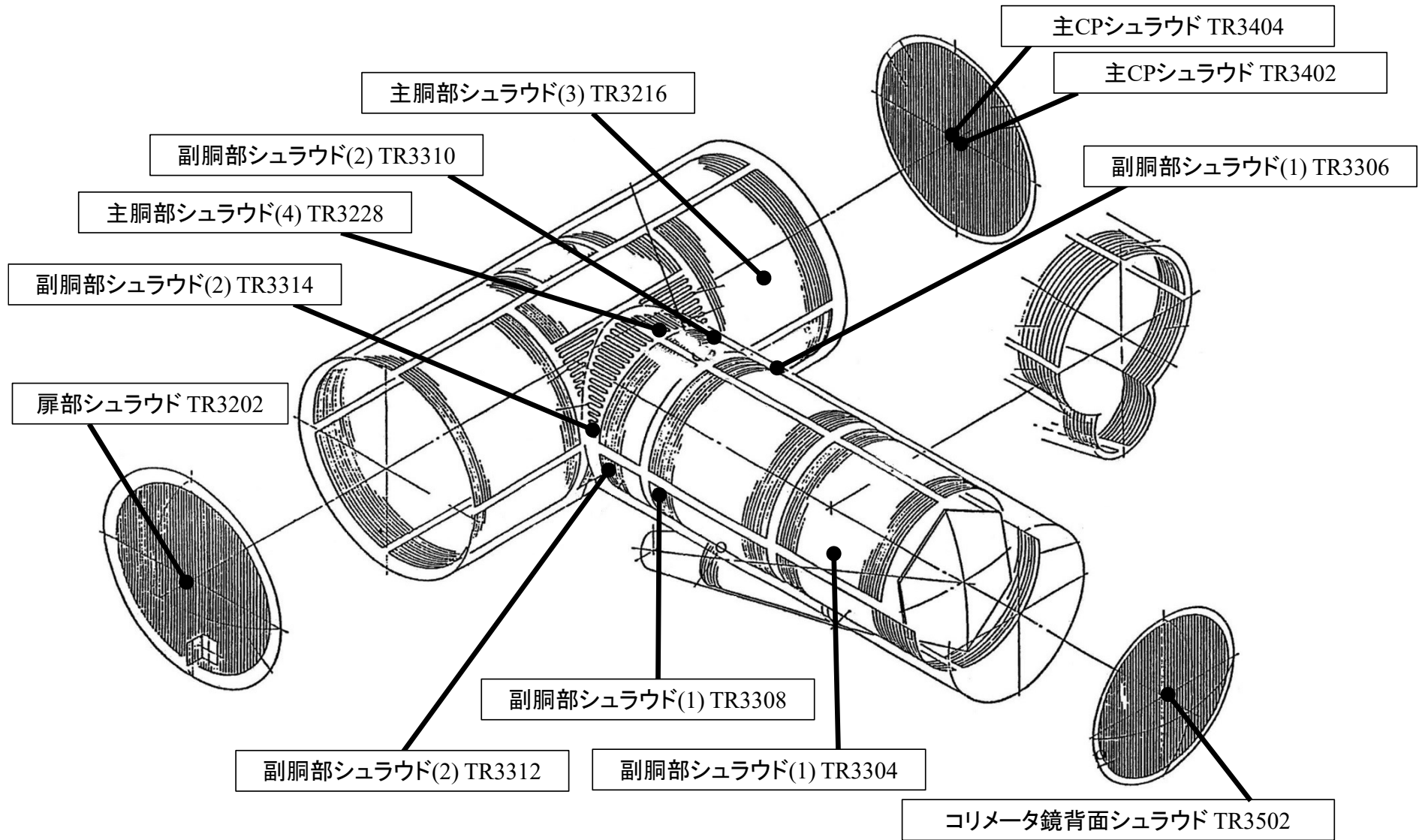
図2-4 シュラウド温度測定位置図 (2/2)
