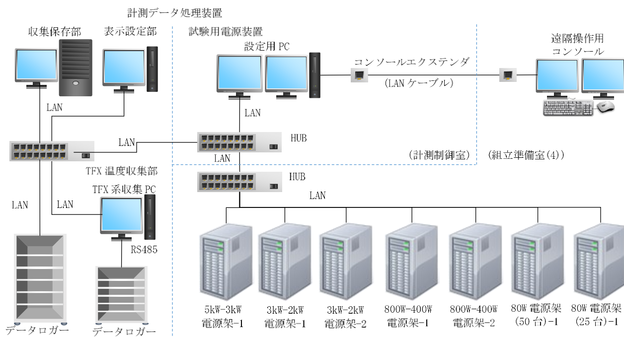
図2-7 試験用電源装置システム構成図
