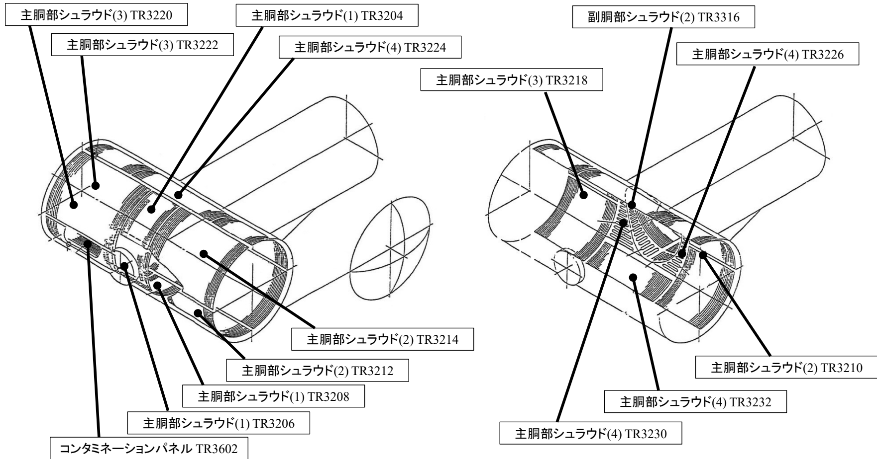
図2-4 シュラウド温度測定位置図 (1/2)
