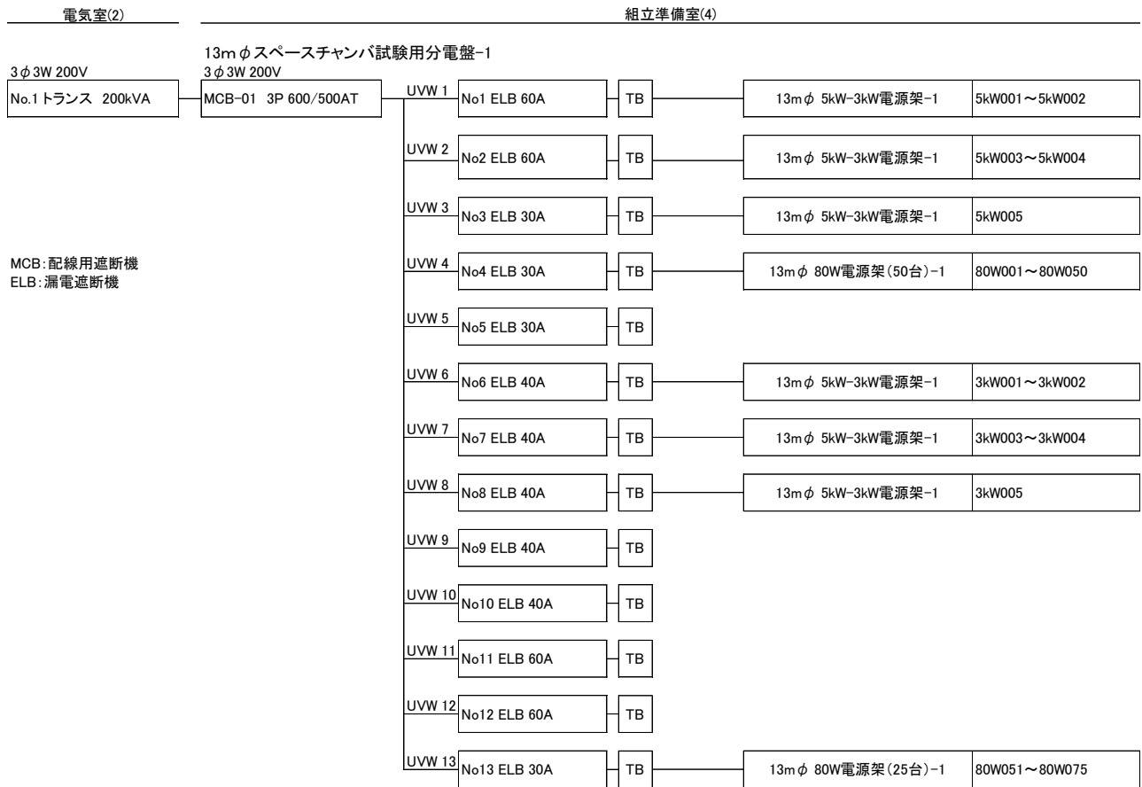
図3-37 試験用電源装置 電源系統図 (1/2)
